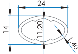
7809 14x24 Elips Profil
