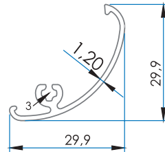
7806 30x30 Elips Profil Kapağı
