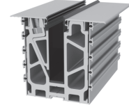
ANC 10-03 Zemin Altı Cam Kanalı Profili (15 cm) Base Profile Built-In 15 cm طقم قاعدي للزجاج تحت الارض 15 سم
