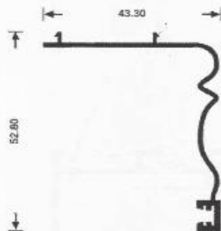
V 160-04 417 gr/m
