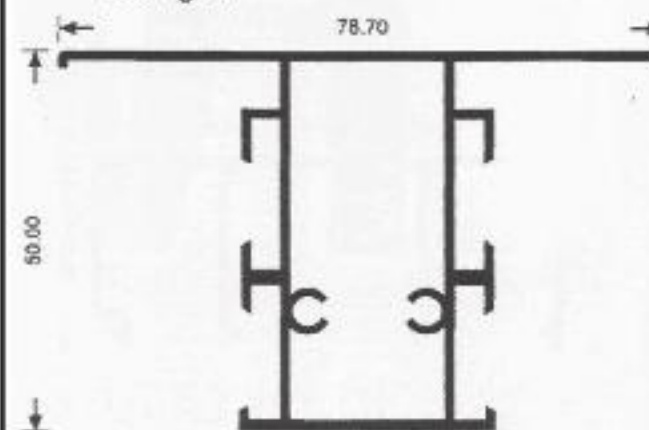
V 120-06 /A 1084 gr/m
