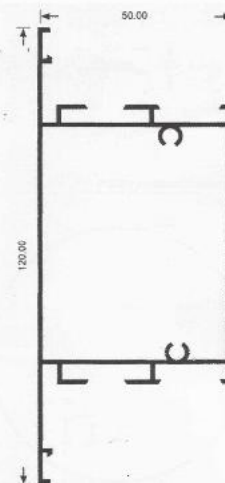
Middle Partitlon V 120-31 1500 gr/m
